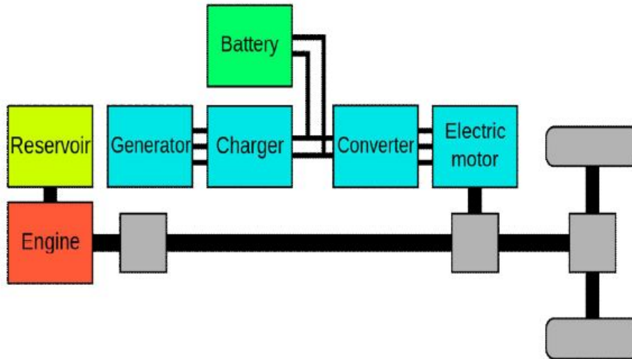
Fig. 5HEV ParallelSeries
